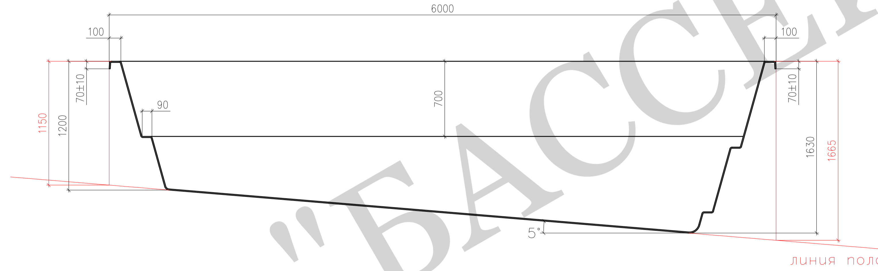
Вид В
