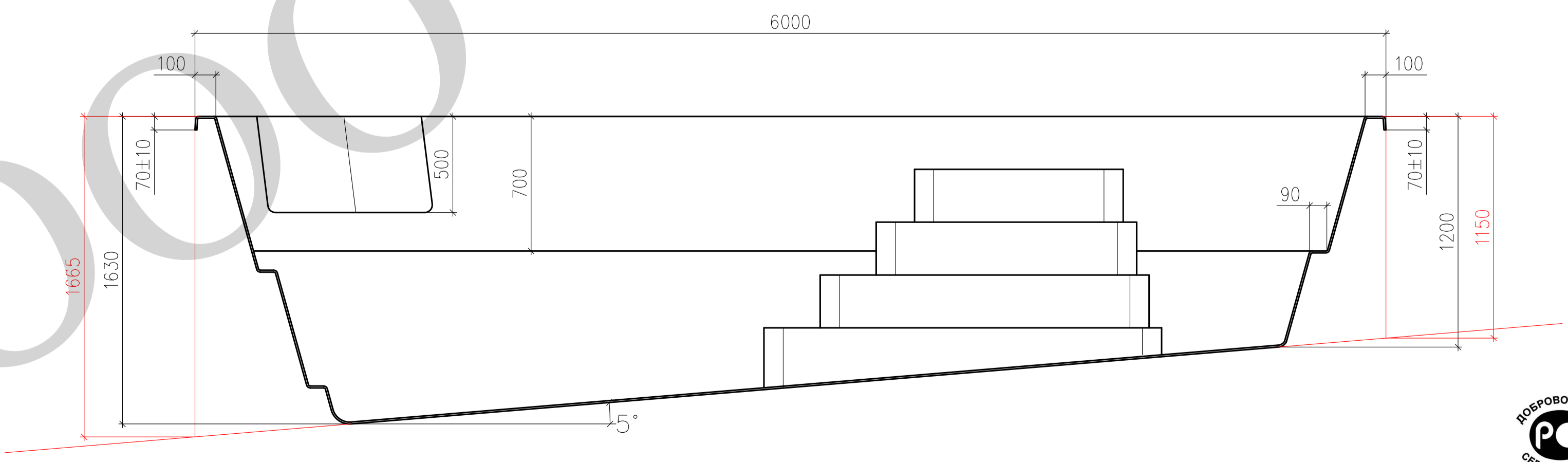
Вид В
